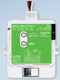
PowPak relay module
