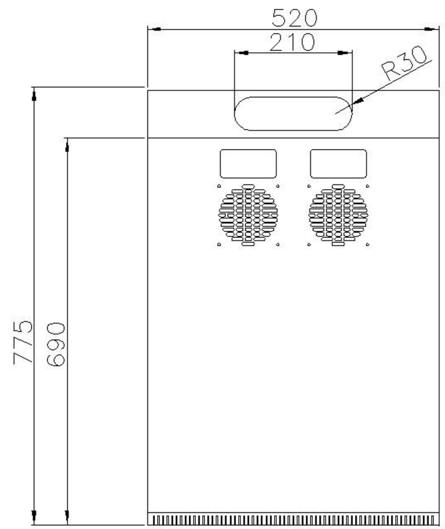
Top
